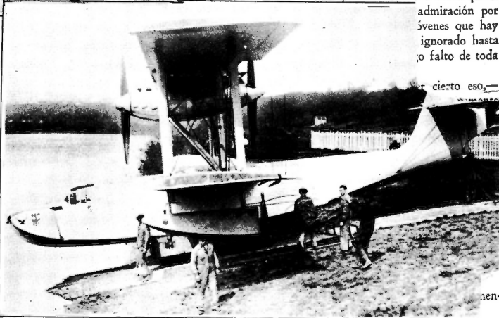
FRANCIA. —El hidroavión gigante, provisto con dos motores de 500 H. P., en que intentarán la travesía del Atlántico, de Este a Oeste, los aviadores franceses teniente Huel y teniente Paris. Los motores, montados en tandem, pueden desarrollar una velocidad de 125 millas por hora.
