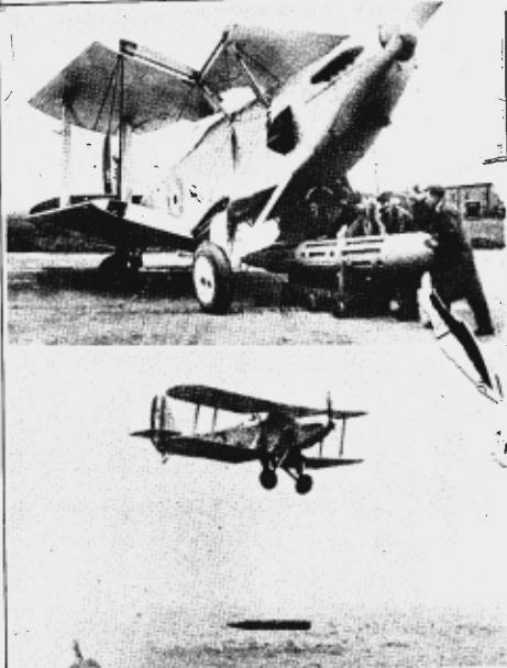
INGLATERRA.—El Ministerio de Aviación inglés ha dotado a sus aviones de un nuevo tipo de torpedo aéreo, que produce un terrible efecto destructor. Este torpedo pesa una tonelada y el avião que lo lleva puede mantenerse con él en el aire durante 12 horas, avanzando a una velocidad de 150 millas.
